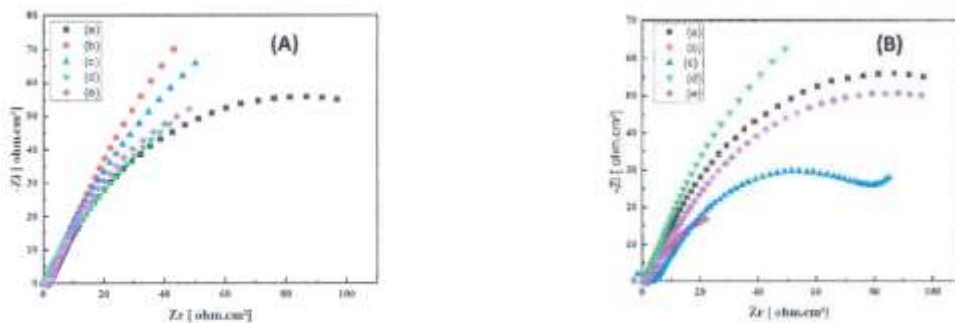
Diagramme d'impédance relative au matériaux composite Pani-MnO 2 (A) et Pani-MgO (B) a différente concentration (a, b, c, d, e) 0,5,10,15 et 20% de MnO 2 et MgO dans une solution de H 2 SO 4 0.5M obtenu sur une gamme de fréquences comprise entre 100 kHz et 10 mHz.
